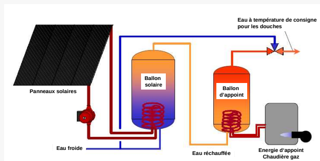
Schéma de principe solaire thermique
